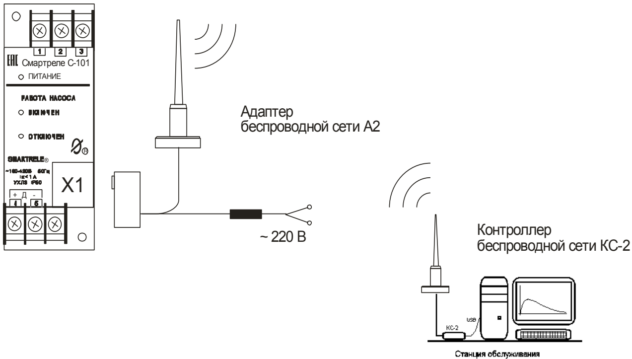
Рисунок 5 – схема подключения реле СМАРТРЕЛЕ C-101, СМАРТРЕЛЕ C-102 к беспроводной сети
