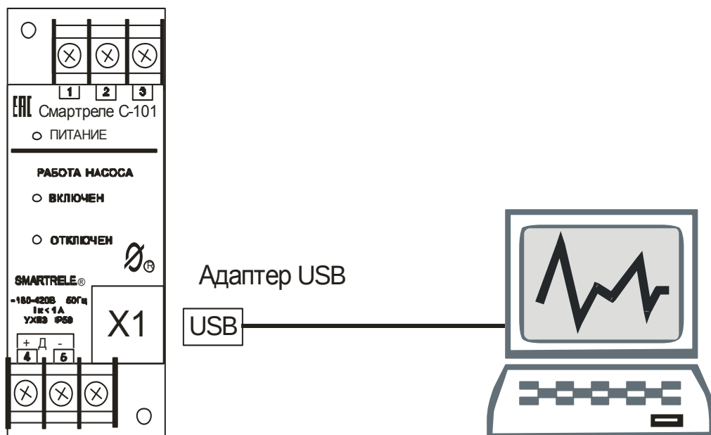
Рисунок 4 – схема подключения реле СМАРТРЕЛЕ C-101, СМАРТРЕЛЕ C-102 к персональному компьютеру (ПК)
